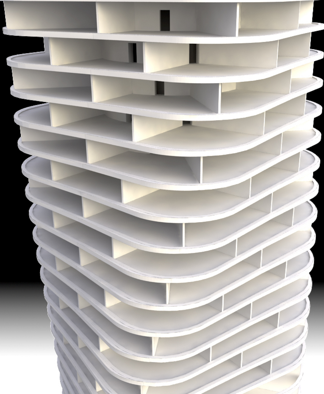
Central Core & Fin Wall Construction
